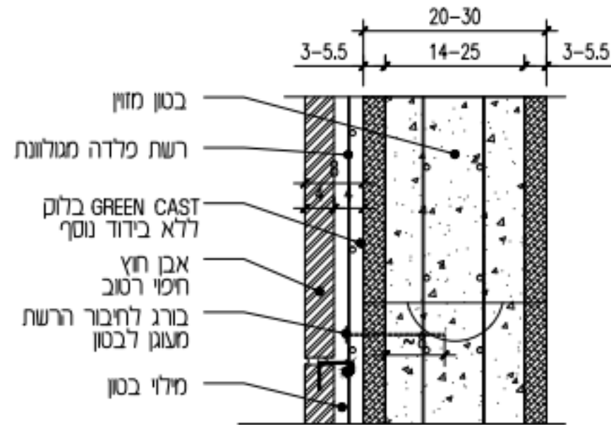
פרט חיפוי אבן על קיר בלוק GREEN CAST בלוק ללא בידוד נוסף תליית אבן בשיטה רטובה
