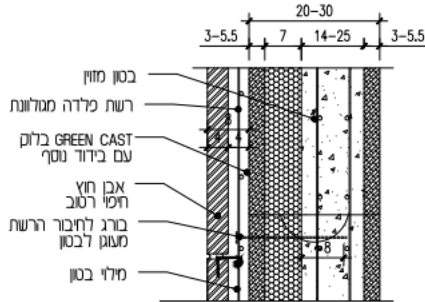
פרט חיפוי אבן על קיר בלוק GREEN CAST בלוק עם בידוד נוסף תליית אבן בשיטה רטובה
